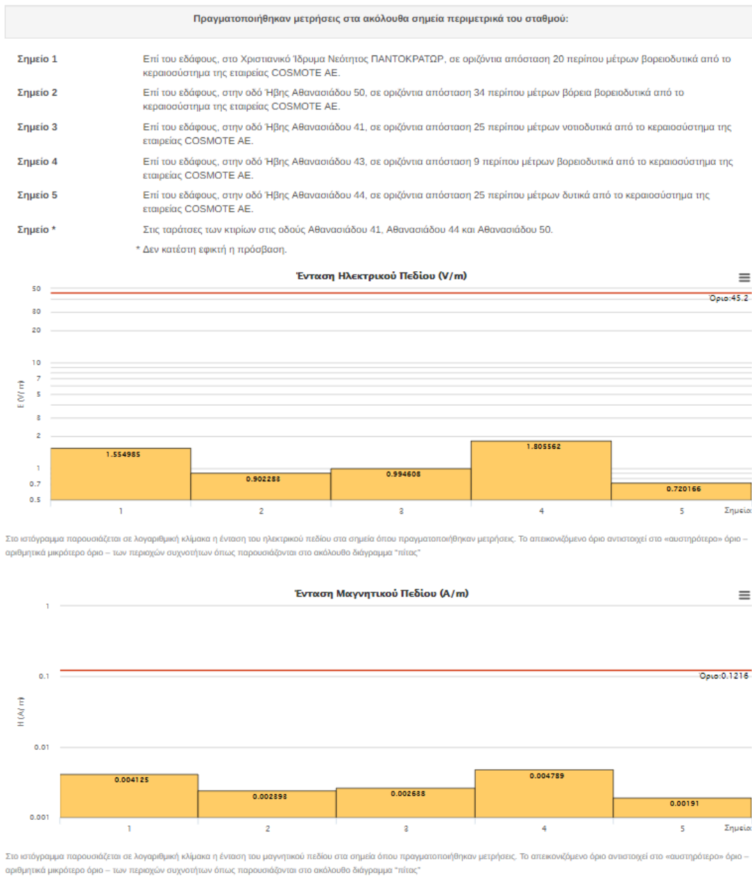
Εικόνα 1: Ενδεικτικές Μετρήσεις Παραμέτρων Ακτινοβολίας μίας Κεραίας [4]
